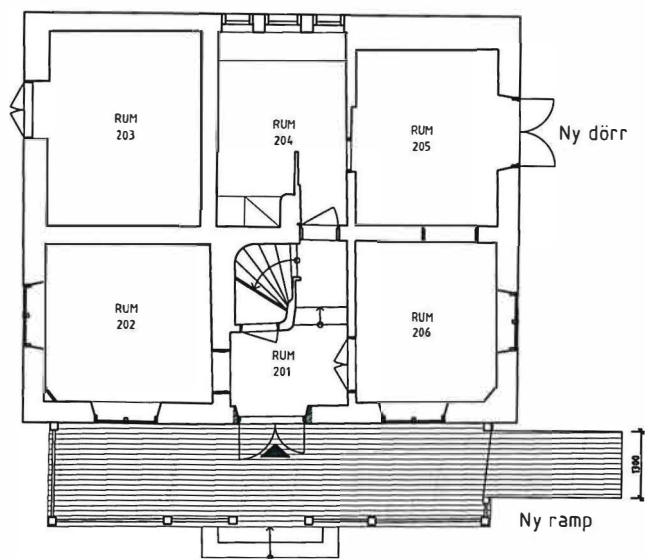
BOTTENVÅNING
