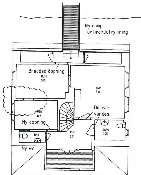
VÅNING 1 TR
